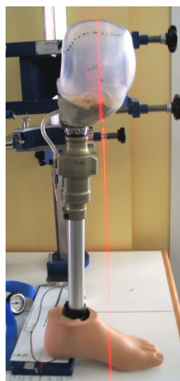
Alignement d'une prothèse transtibiale
